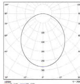
Levanto R LED1x1050 B251 T840 L80 Levanto R LED1x1050 B288 T840 L80
