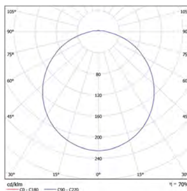
Eta LED1x1050 B680 T840
