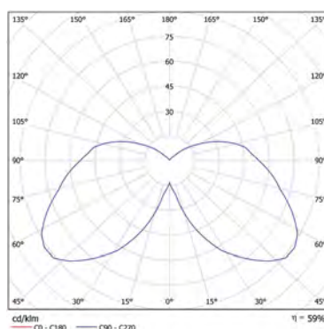
Sargas 1E27 N68 CLR RFL ROOF
