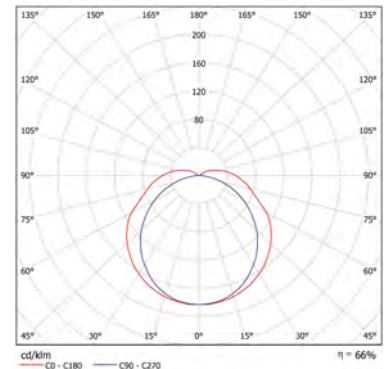
Star 236 001 PRZ HF
