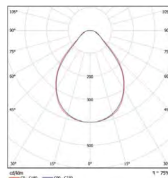
Marengo R LED1x1050 B269 T840 Marengo R LED2x2000 B273 T840
