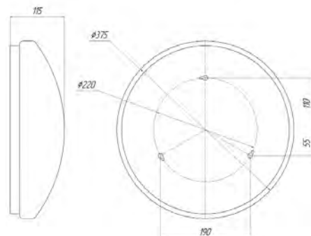
Pavo 2E27 M47
