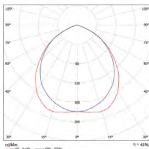
Orion 218 B27 OP
