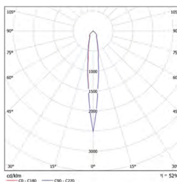
Radius 135 N81 HI
