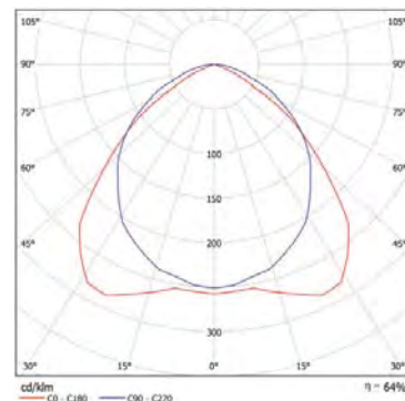
Passat 418 A30 HF
