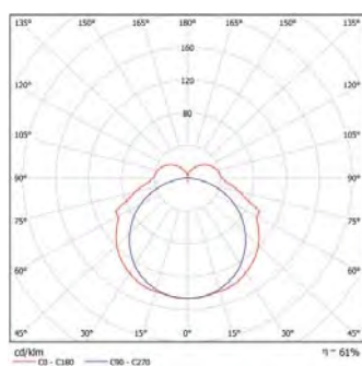
Euros 258 H12 OP HF
