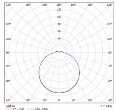
Dorado B 218 H30
