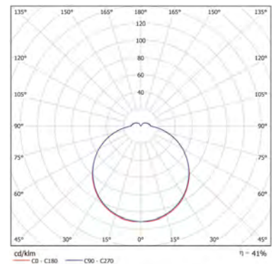
Dorado 109 H27 HF
