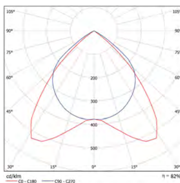
Decor D 228 M89 PAR
