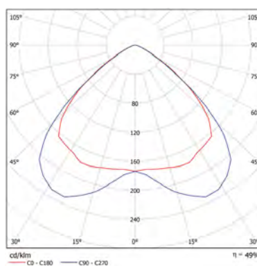
Orion 218 B27 MIR
