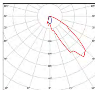
Arena 11000 N86 BLD
