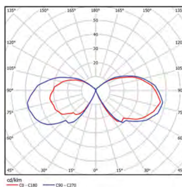
Draco 132 N64 HF
