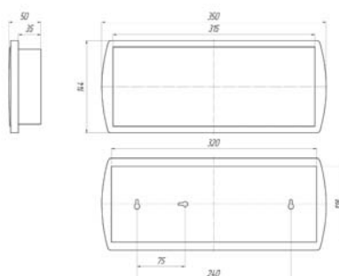
Vega 1H18 B73
