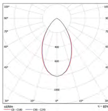
Radius LED1x2500 B651 T750 L60
