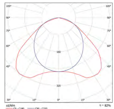
Alcor 228 A59 DeLuxe
