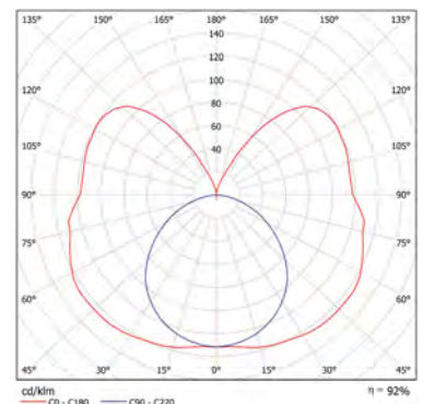
Bora 136 A73 HF
