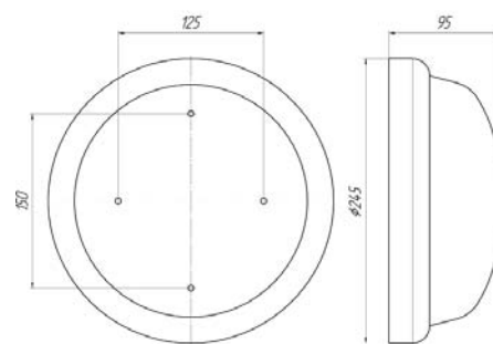
Circus 113 J53 OP
