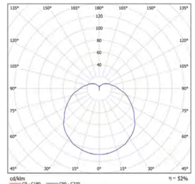
Pavo 232 O49 HF
