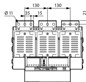
Задние выводы
