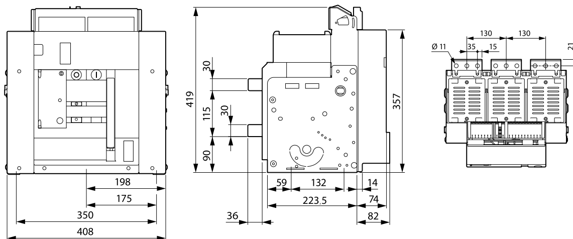
Задние выводы
