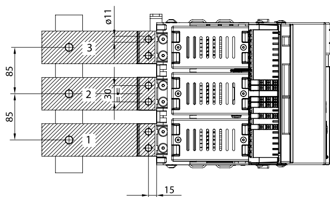
ПРОТОН 25 Nord
