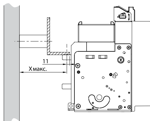
ПРОТОН 40 Nord
