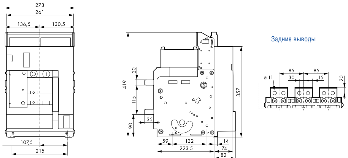
Задние выводы
