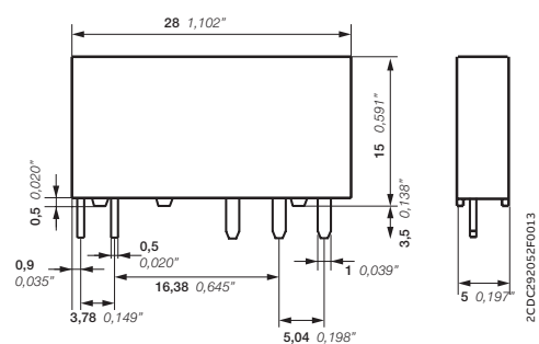
Реле CR-S
