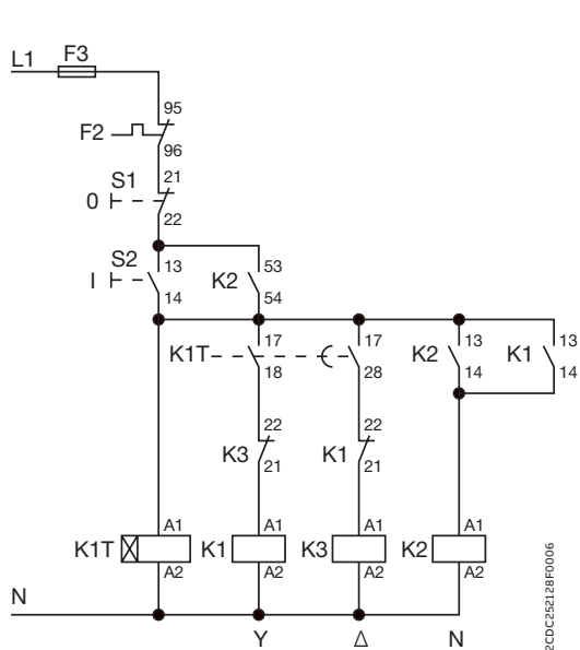
Схема цепи управления
