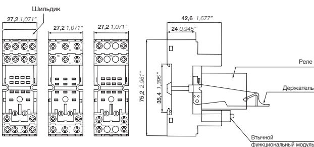
CR-M2SS — CR-M3SS — CR-M4SS с винтовыми клеммами
