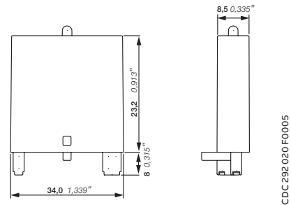
Функциональный модуль CR-Uxx
