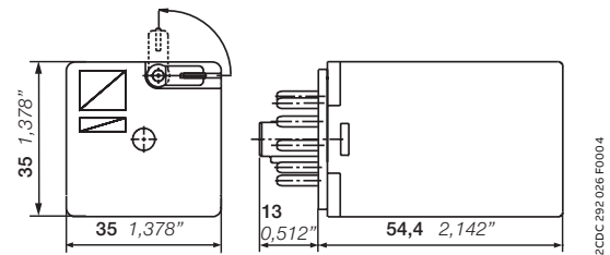
Реле CR-U с 3 переключающими контактами
