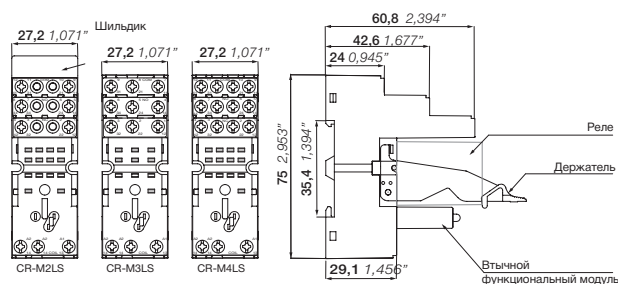
CR-M2LS — CR-M3LS — CR-M4LS с винтовыми клеммами
