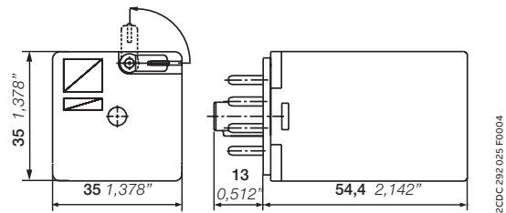
Реле CR-U с 2 переключающими контактами
