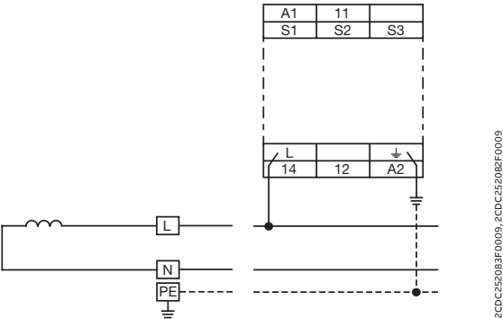
2-проводная сеть переменного тока
