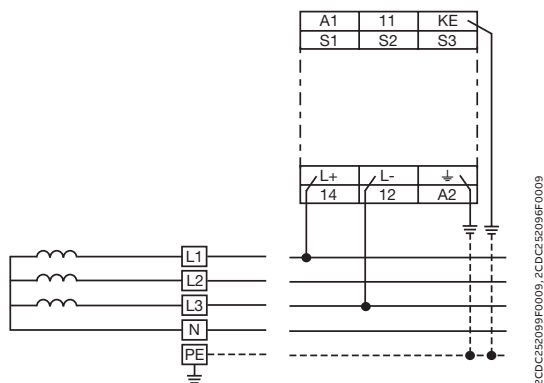
4-проводная сеть переменного тока
