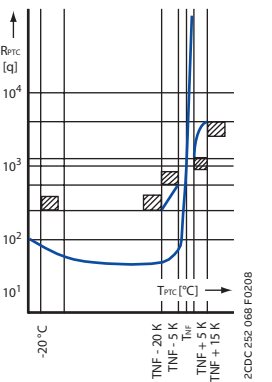
Характеристики термисторного датчика (РТС)
