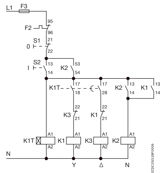
Схема цепи управления
