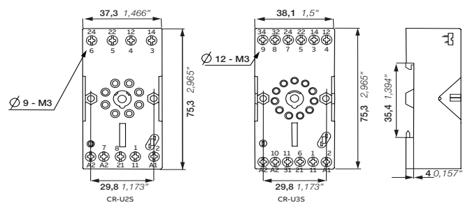
CR-U25 — CR-U35 с винтовыми клеммами
