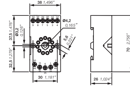
CR-U3E с винтовыми клеммами
