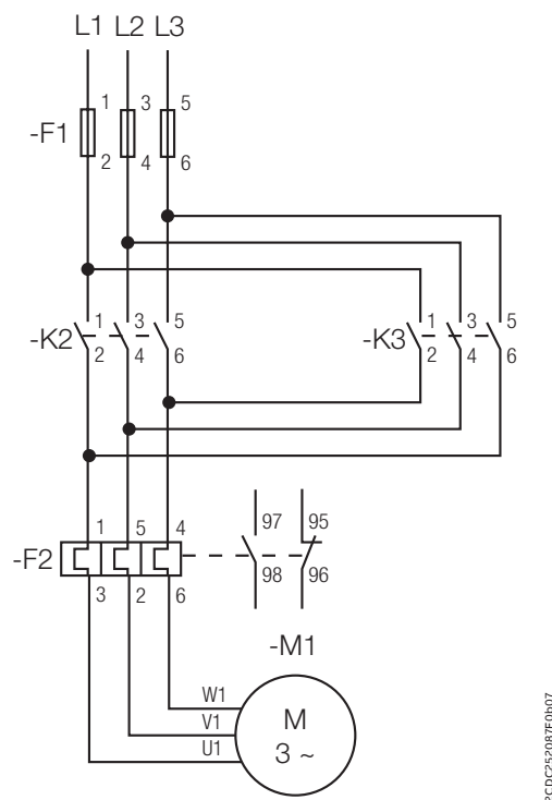
Схема силовой цепи
