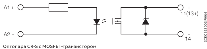
Оптопара CR-S с MOSFET-транзистором
