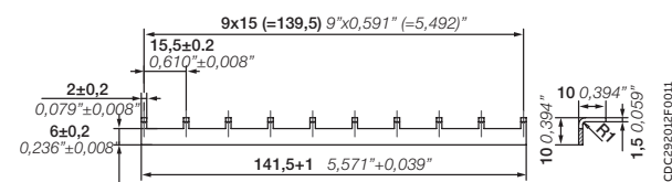
Перемычка CR-PJ
