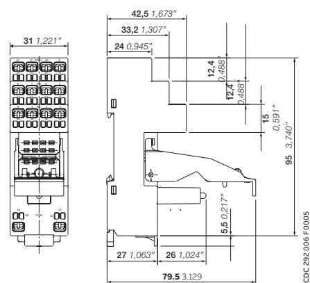
CR-M2LC, CR-M4LC с пружинными клеммами
