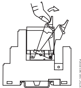
Демонтаж
