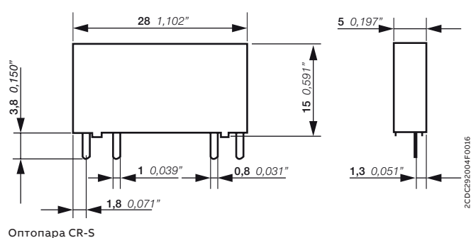
Оптопара CR-S
