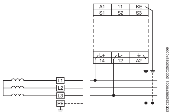
3-проводная сеть переменного тока
