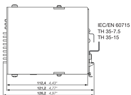
CP-B 24/3.0
