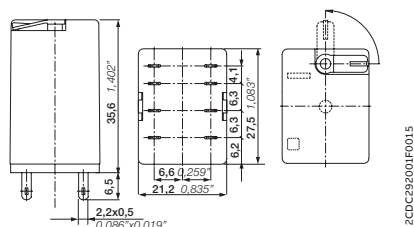
Реле CR-M с 2 переключающими контактами
