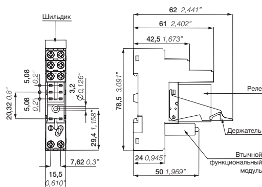
CR-PLSx с винтовыми клеммами
