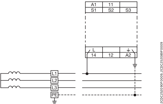
3-проводная сеть переменного тока
