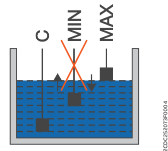
Режим работы с двумя электродами
