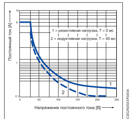
CR-M с 4 переключающими контактами
