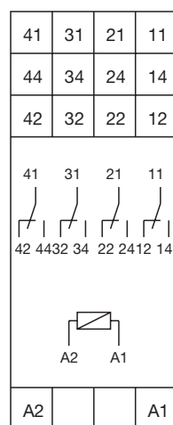
CR-M4LC
