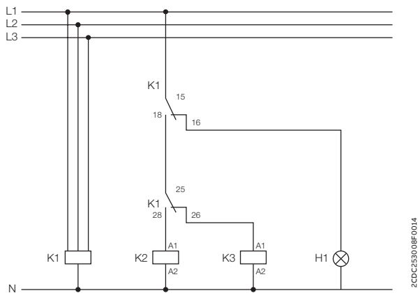
Схема цепи управления (К1 = СМ-МПС.23)
