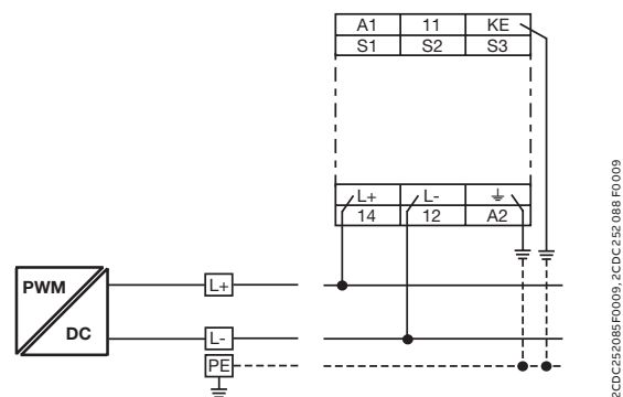
2-проводная сеть постоянного тока
