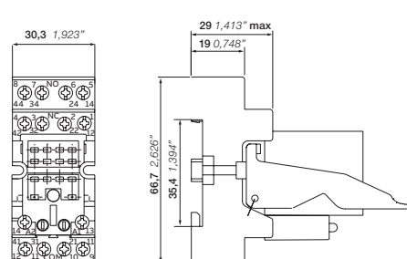
CR-MxSF с винтовыми клеммами
