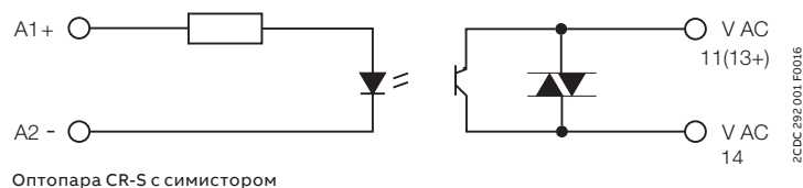
Оптопара CR-S с симистором
