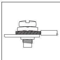
07 Вилочное соединение
