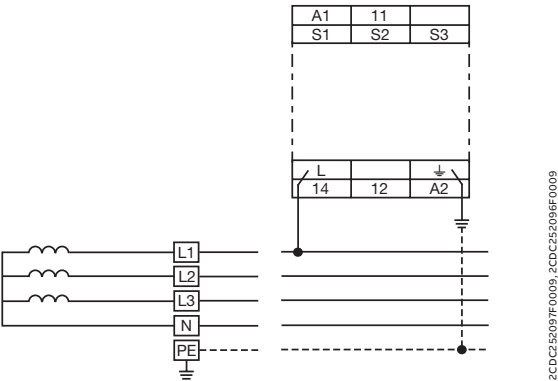
4-проводная сеть переменного тока
