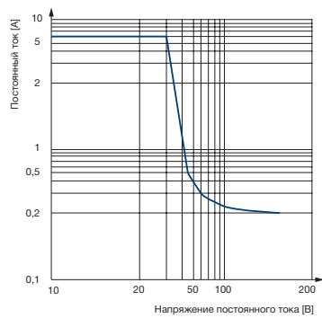
Макс. отключающая способность, нагрузка DC
