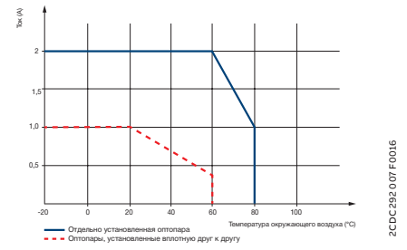
Выход CR-S с симистором
