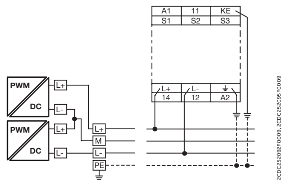
3-проводная сеть постоянного тока
