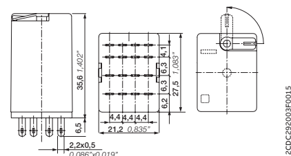
Реле CR-M с 4 переключающими контактами
