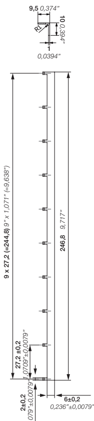
Перемычка CR-MJ
