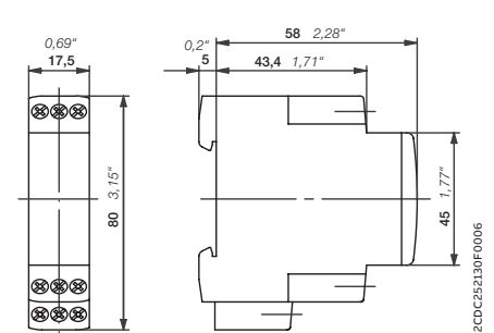
Устройства СТ-D с 2 переключающими контактами
