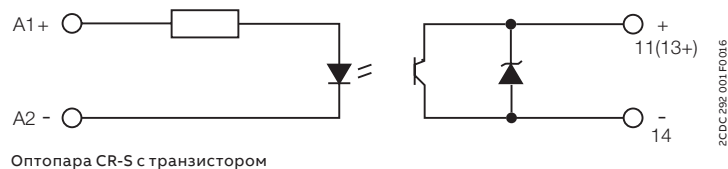
Оптопара CR-S с транзистором
