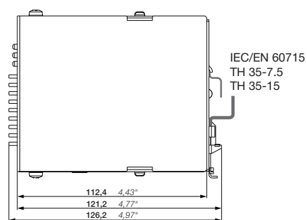
CP-B EXT.2
