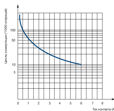
Кривая износоустойчивости
