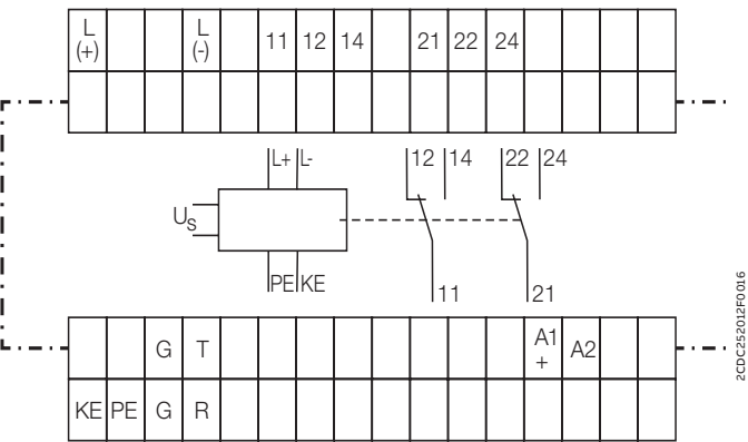
СМ-IWM.10
