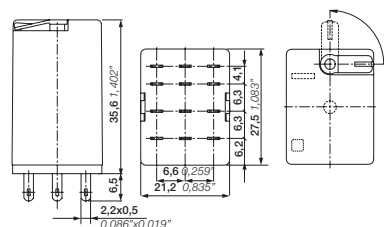
Реле CR-M с 3 переключающими контактами
