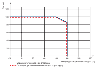
Транзисторный выход CR-S
