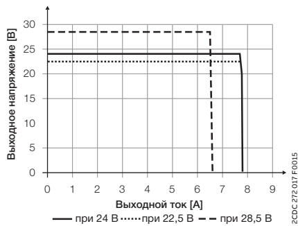
CP-C.1 24/5.0
