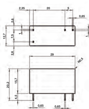
Оптопара CR-P
