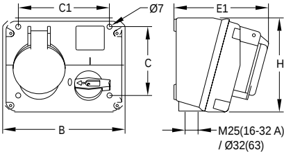
Габаритные размеры (мм)
